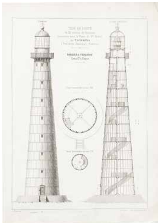
Tuletorni joonis Barbier & Fenestre „Tour en fonte de Tachkona“. ParisTech archive École des Ponts. Foto: Indrek Laos
